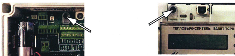
Рисунок 3 – Места пломбировки от несанкционированного доступа тепловычислителей ВЗЛЕТ ТСРВ
